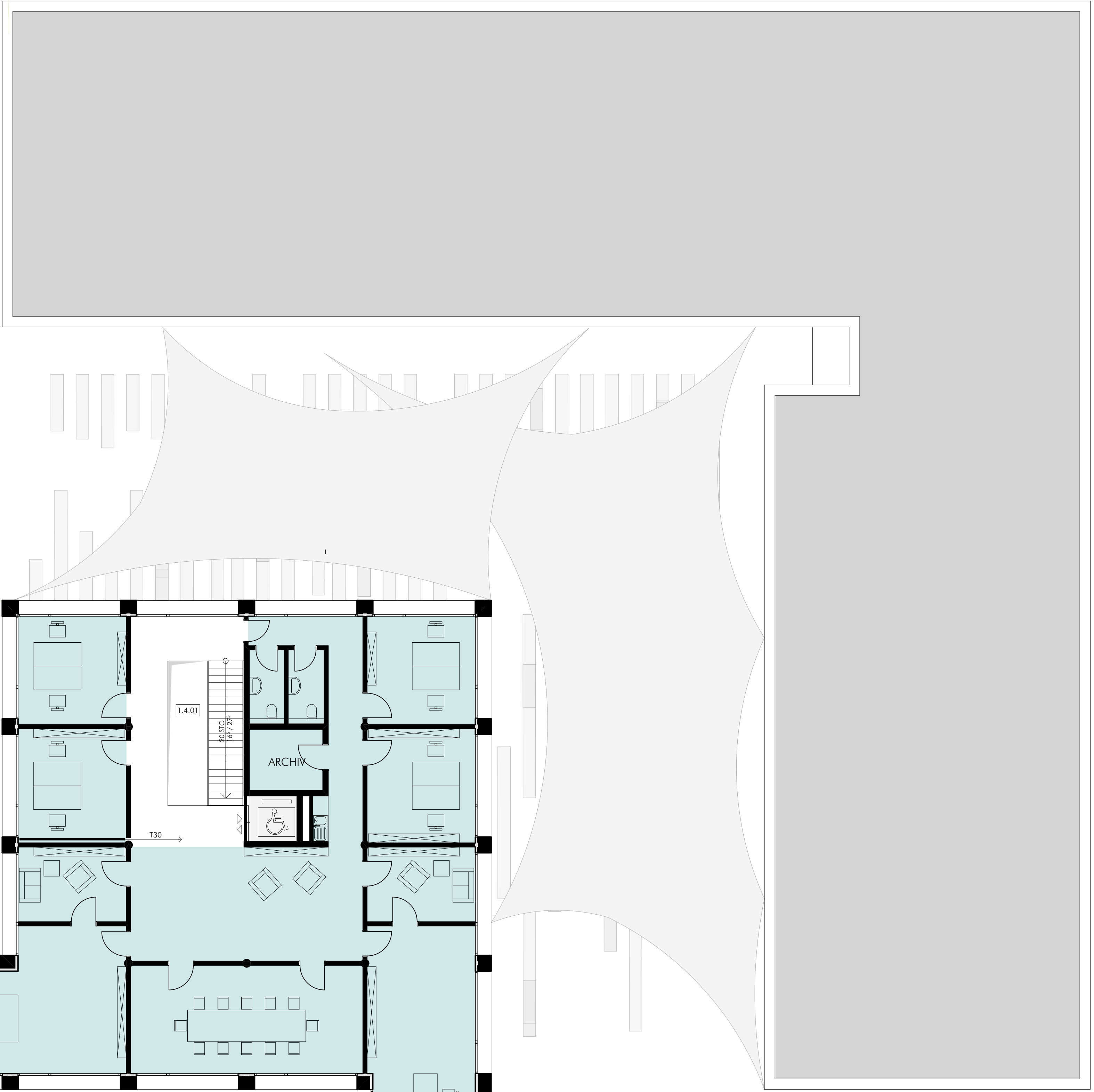
GRUNDRISS 4. OBERGESCHOSS
